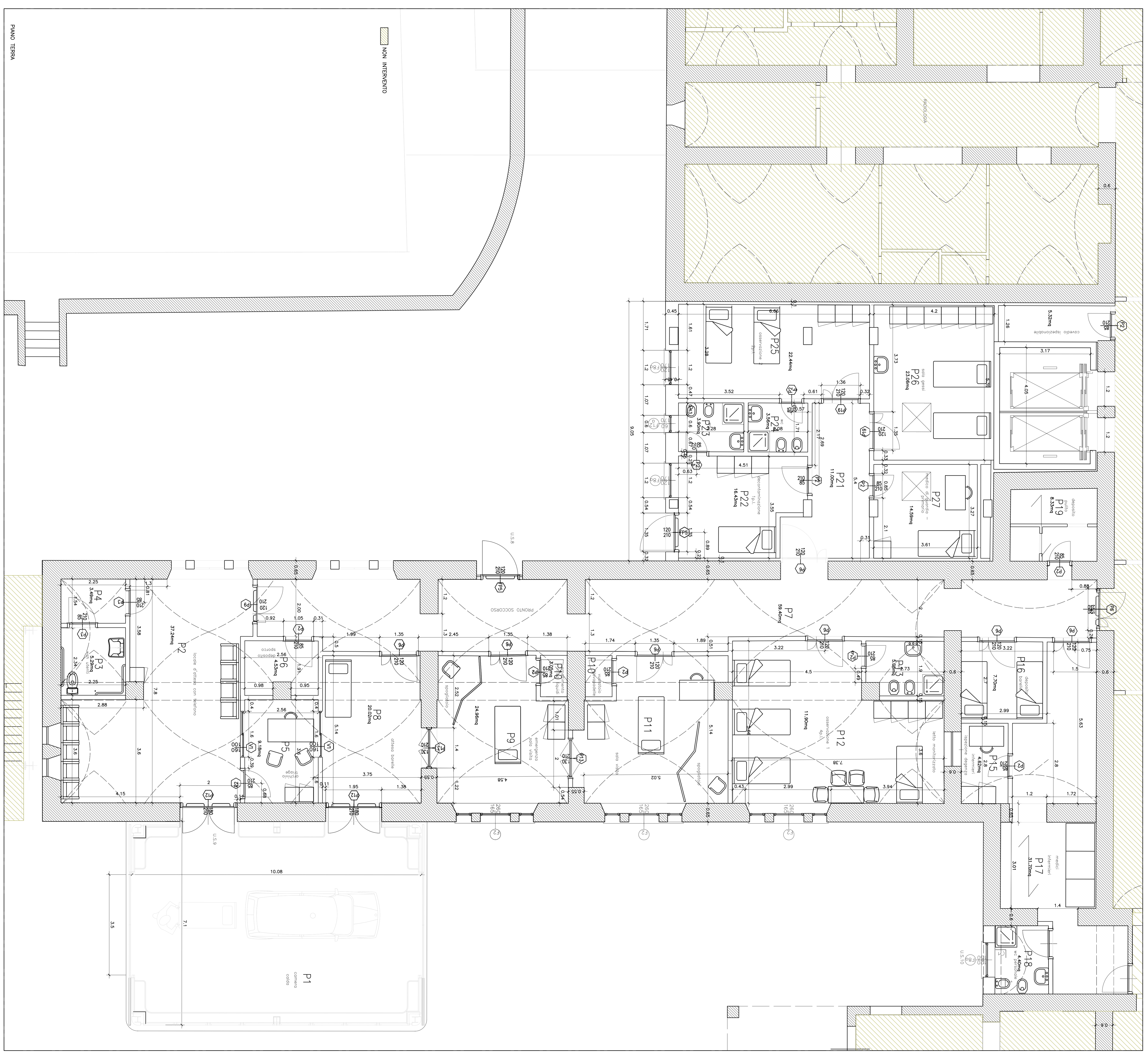
PIANO SOTTOTETTO
